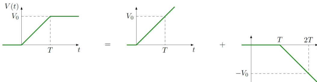
Consigne de vitesse de déplacement d'un ascenseur
