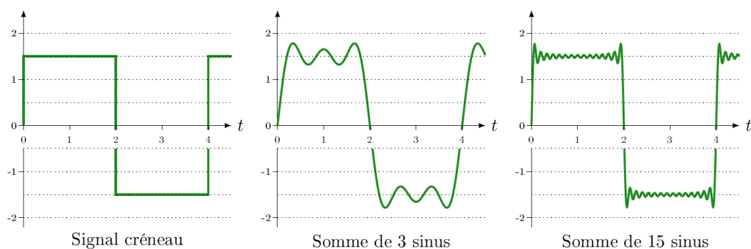
Décomposition en série de Fourier d'un signal créneau
